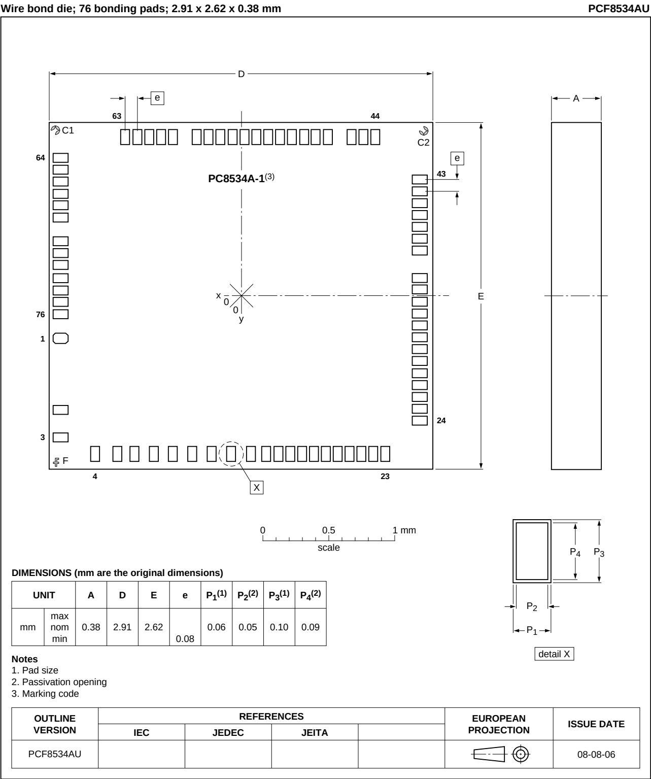
Fig 26. PCF8534AU die outline
